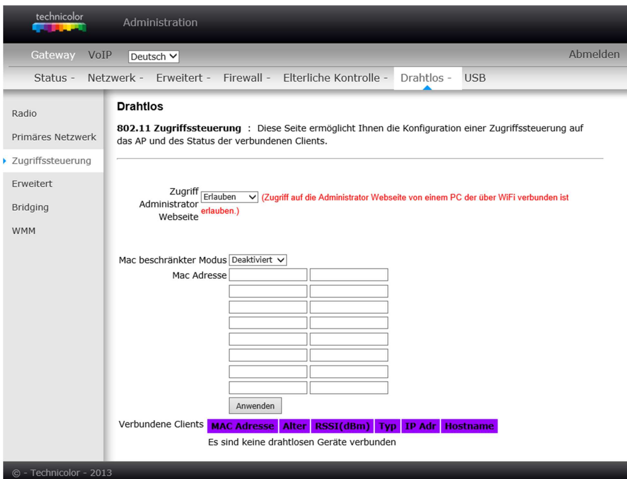
Abb. 2-38 Gateway\Drahtlos\Zugriffssteuerung
