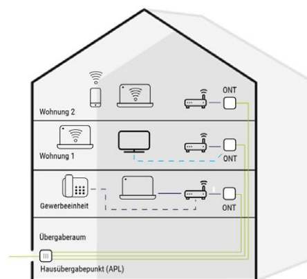
APL im Keller + ONT und Router in jeder Wohnung
