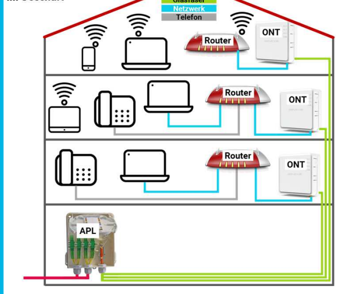
Haus mit div. WE/GE ONT in der Wohnung / im Geschäft
