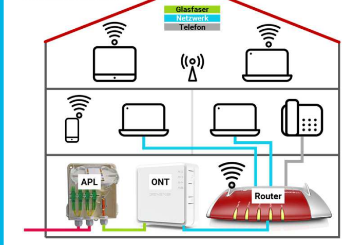
Haus mit einer WE/GE ONT im Anschlussraum
