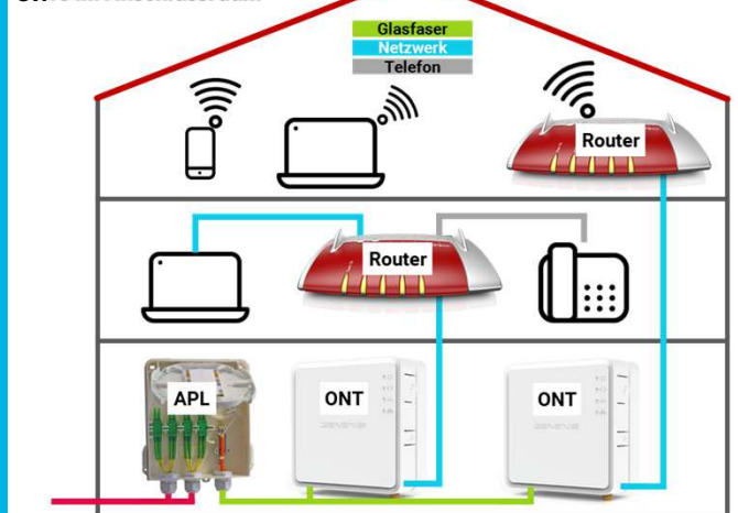
Haus mit zwei WE/GE ONTs im Anschlussraum
